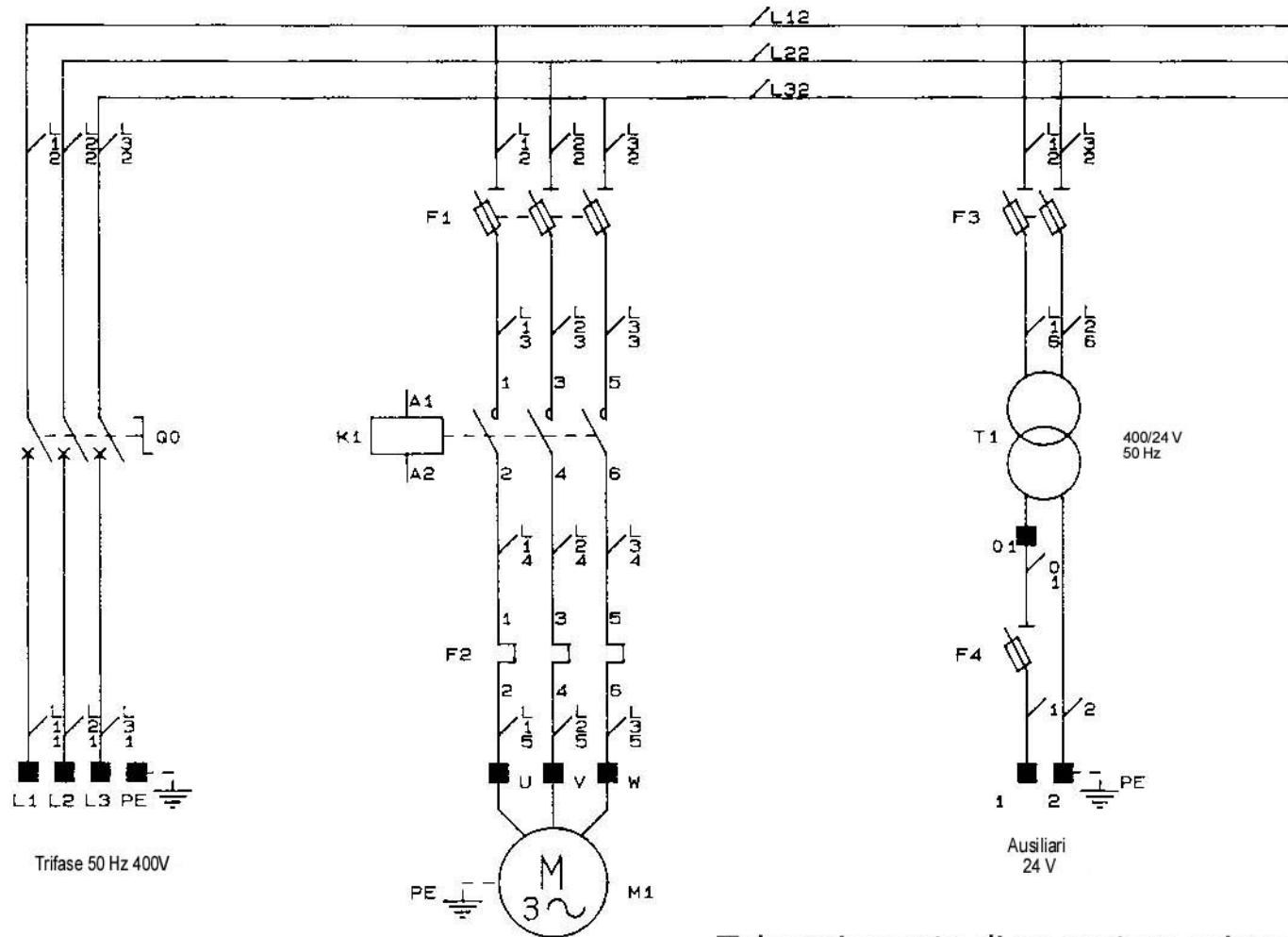
Teleavviamento di un motore asincrono trifase
